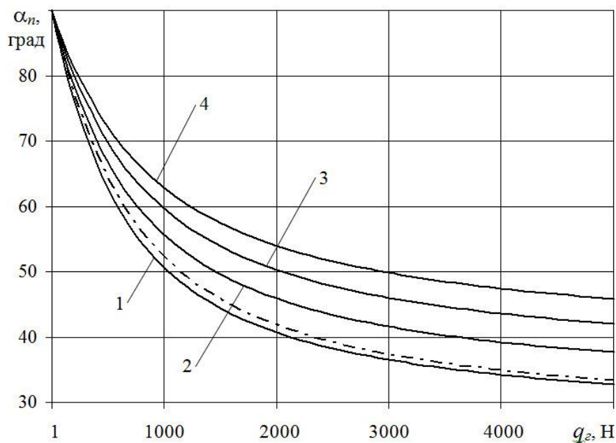
Рисунок 2 – График зависимости предельного угла наклона ленточного конвейера с прижимной лентой \alpha_n от погонной q_2 при различных значениях коэффициента трения груза о ленту f_1
