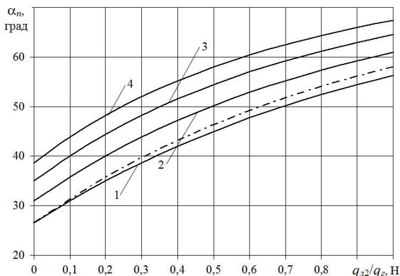
Рисунок 3 – График зависимости предельного угла наклона ленточного конвейера с прижимной лентой \alpha_n от отношения погонного веса прижимной ленты q_{л2} к погонному весу груза q_z при различных значениях коэффициента трения груза о ленту f_1
